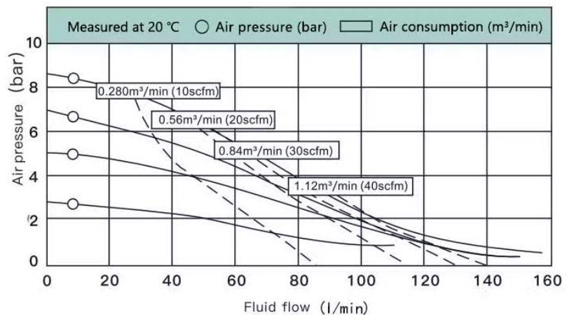
Curvas de rendimiento del KES25
